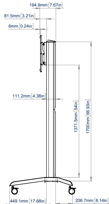
VUE LATÉRALE
