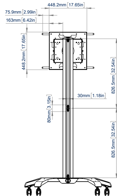
VUE ARRIÈRE
