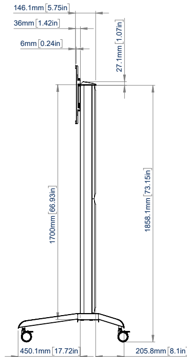
VUE LATÉRALE
