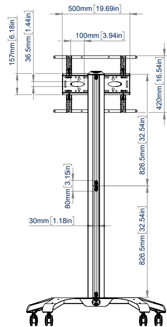
VUE ARRIÈRE
