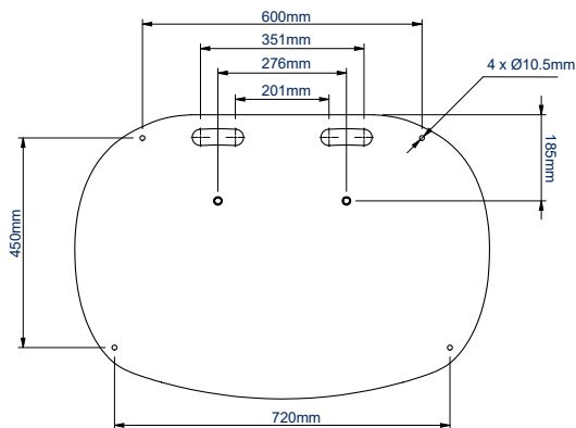
VUE BASE
