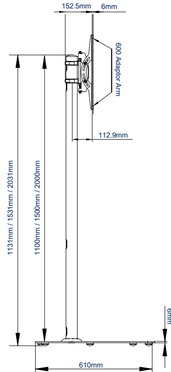
VUE LATÉRALE
