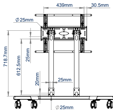
VUE ARRIÈRE
