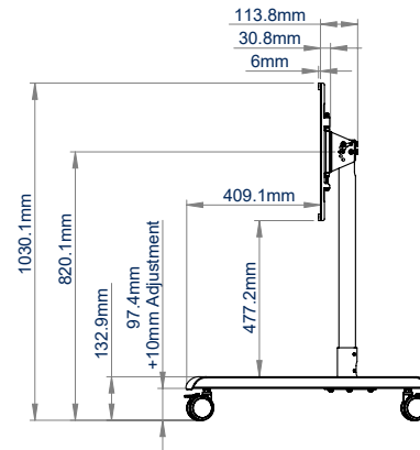
VUE LATÉRALE
