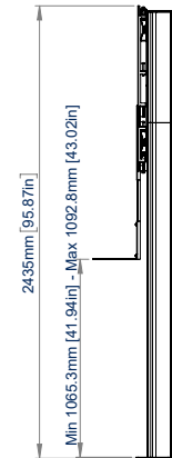
VUE LATÉRALE
