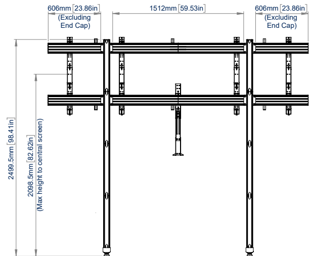
VUE ARRIÈRE
