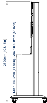
VUE LATÉRALE
