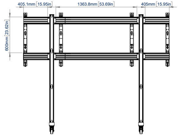
VUE ARRIÈRE
