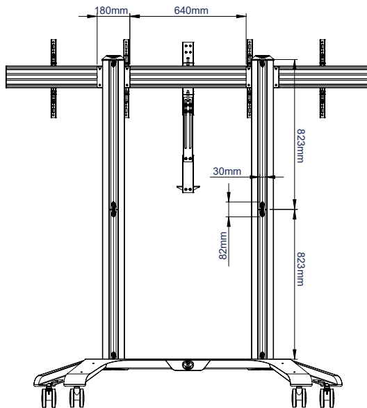
VUE ARRIÈRE
