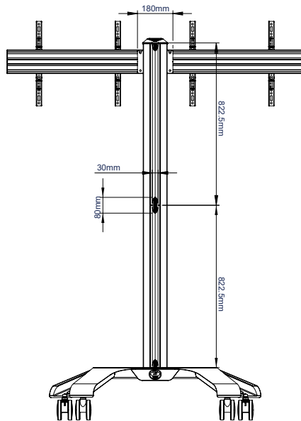
VUE ARRIÈRE
