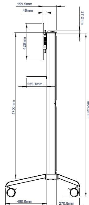
VUE LATÉRALE
