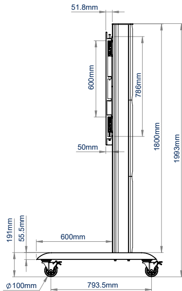
VUE LATÉRALE
