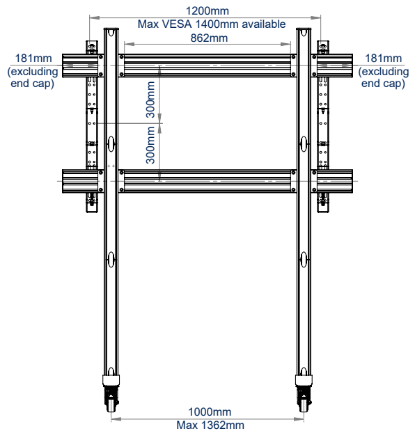
VUE ARRIÈRE
