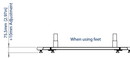
VUE DE FACE PIEDS RÉGLABLES
