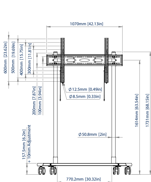
VUE DE FACE AVEC CASTORS
