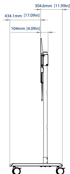
VUE LATÉRALE AVEC CASTORS
