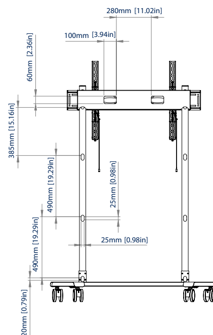
VUE ARRIÈRE AVEC CASTORS
