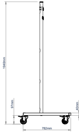
VUE LATÉRALE AVEC CASTORS
