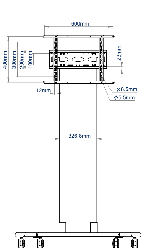
VUE DE FACE AVEC ROULETTES
