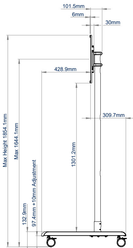
VUE LATÉRALE AVEC ROULETTES
