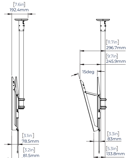
VUE LATÉRALE
