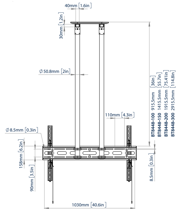
VUE ARRIÈRE
