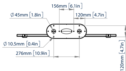
PLAQUE DE PLAFOND VUE DE DESSUS
