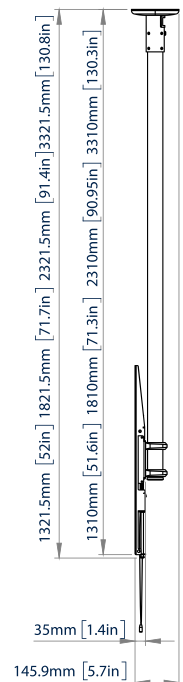
VUE LATÉRALE
