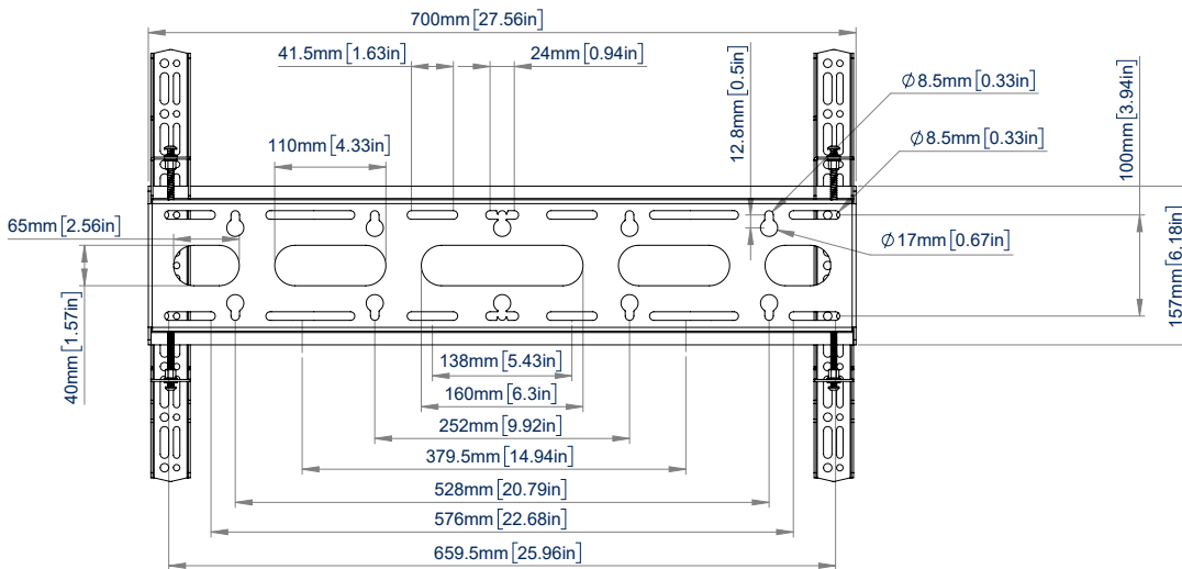
VUE ARRIÈRE
