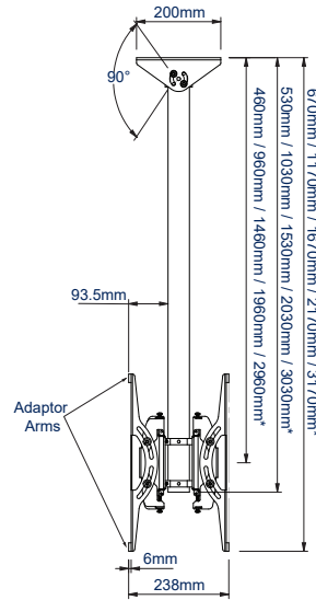
VUE LATÉRALE INTERFACE PLATE
