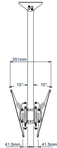
VUE LATÉRALE INCLINAISON DE L'INTERFACE VERS LE BAS
