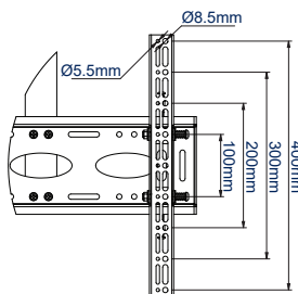
INTERFACE ARM VUE EN GROS PLAN
