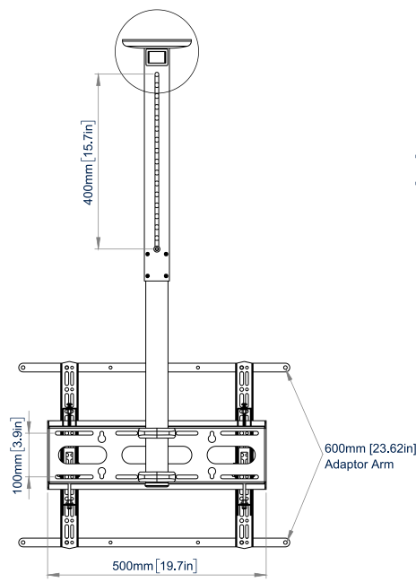
VUE ARRIÈRE
