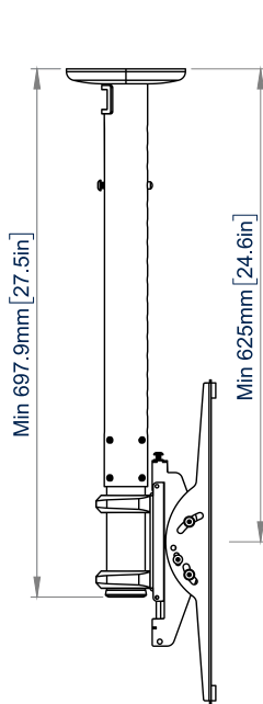
VUE LATÉRALE MIN EXTENSION
