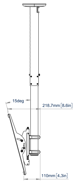
VUE LATÉRALE AVEC INCLINAISON
