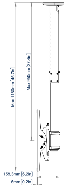
VUE LATÉRALE MAX EXTENSION
