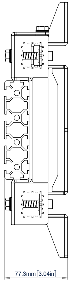
VUE LATÉRALE AVEC BT8390 RAIL DE MONTAGE PROFONDEUR MAXIMALE
