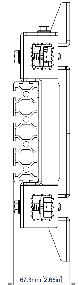
VUE LATÉRALE
