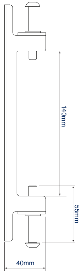
VUE LATÉRALE
