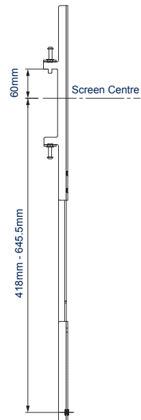
VUE LATÉRALE AVEC BARRE D'EXTENSION - RAIL INFÉRIEUR
