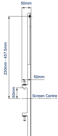
VUE LATÉRALE RAIL SUPÉRIEUR
