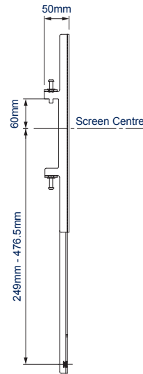
VUE LATÉRALE SOUS LE RAIL
