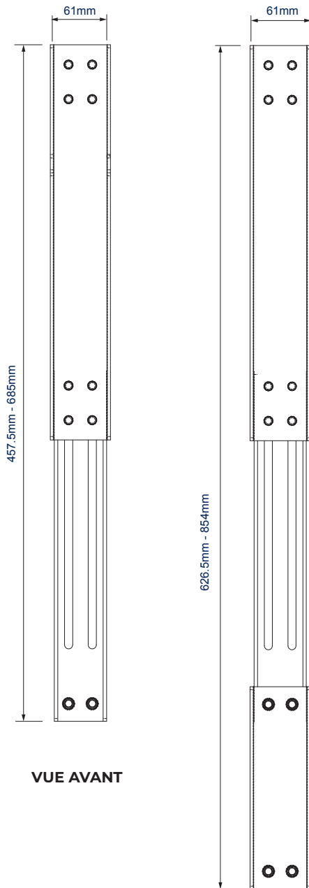
VUE DE FACE AVEC BARRE D'EXTENSION
