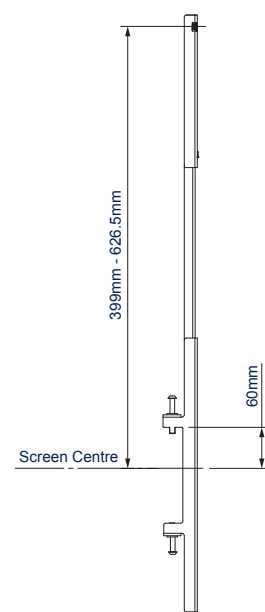
VUE LATÉRALE AVEC BARRE D'EXTENSION - RAIL SUPÉRIEUR
