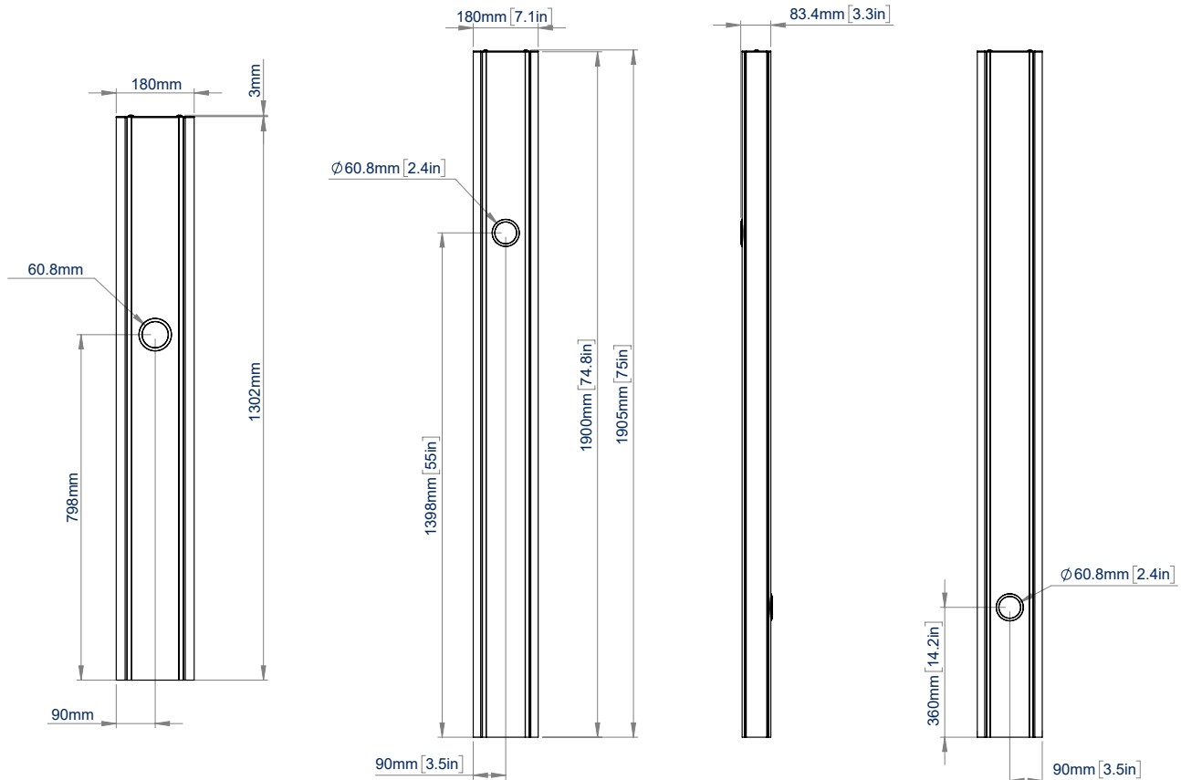
BT8385-130 VUE DE FACE
