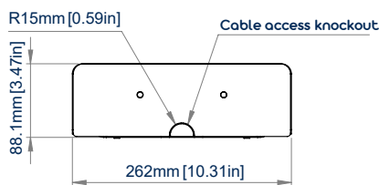
VUE ARRIÈRE
