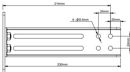
VUE LATÉRALE - PLAQUE DE CONNEXION
