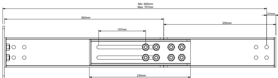
VUE LATÉRALE - PLAQUE DE CONNEXION AVEC PLAQUE D'EXTENSION LONGUE
