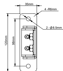
VUE DE FACE - PLAQUE MURALE
