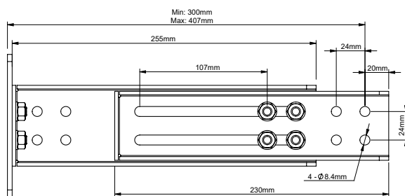
VUE LATÉRALE - PLAQUE DE CONNEXION AVEC PLAQUE D'EXTENSION COURTE
