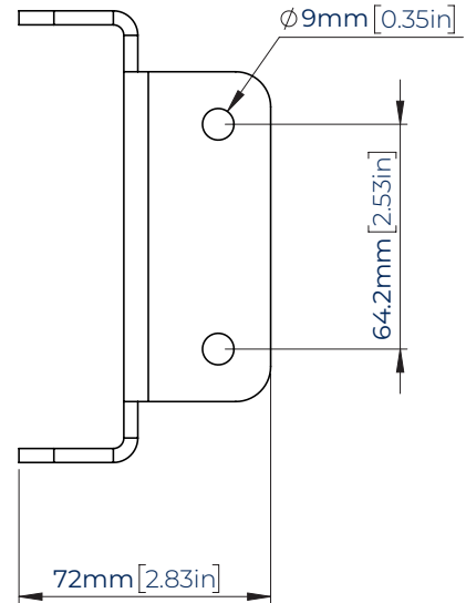
VUE LATÉRALE
