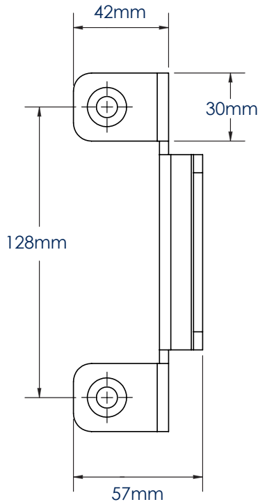
VUE LATÉRALE
