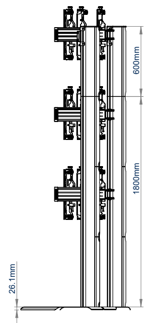
VUE LATÉRALE
