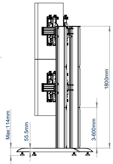
VUE LATÉRALE
