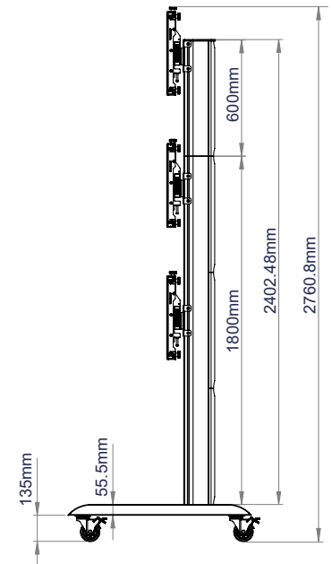
VUE LATÉRALE
