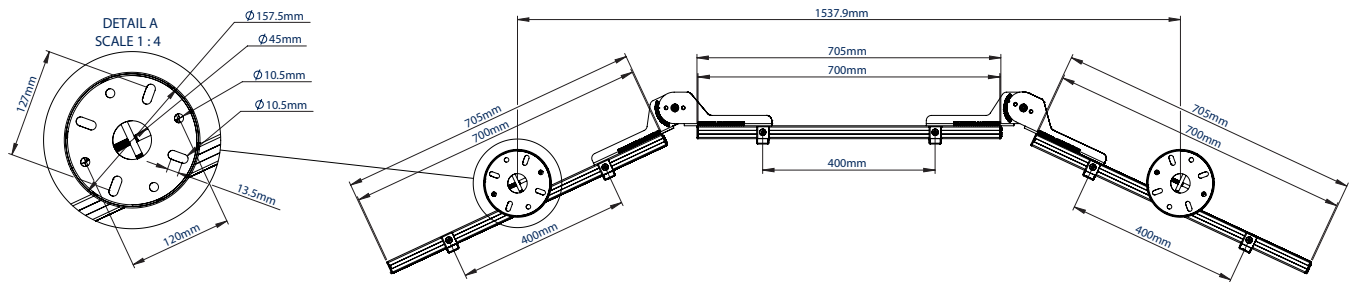
VUE DU DESSUS (PLAQUE DE PLAFOND)
