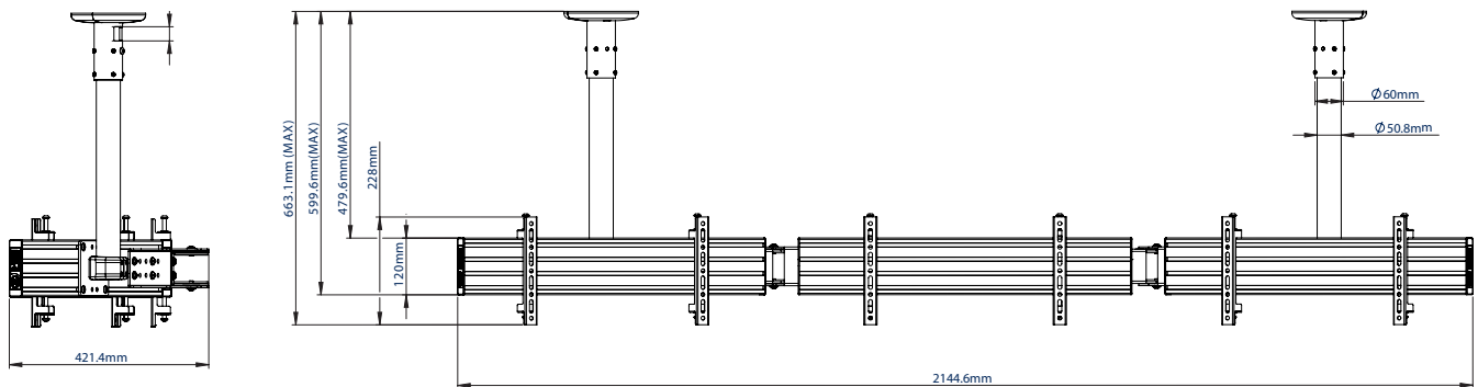
VUE LATÉRALE
