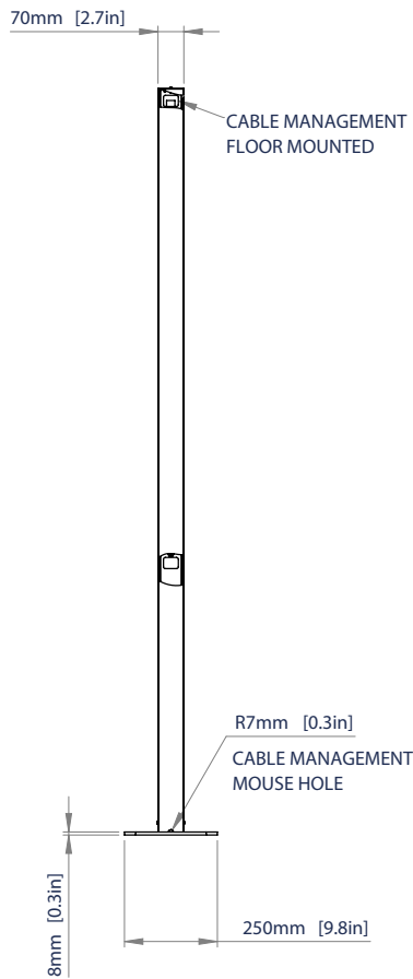
VUE LATÉRALE
