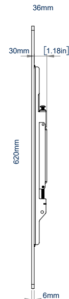
VUE LATÉRALE
