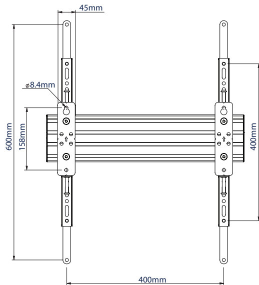
VUE ARRIÈRE
