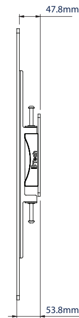
VUE LATÉRALE
