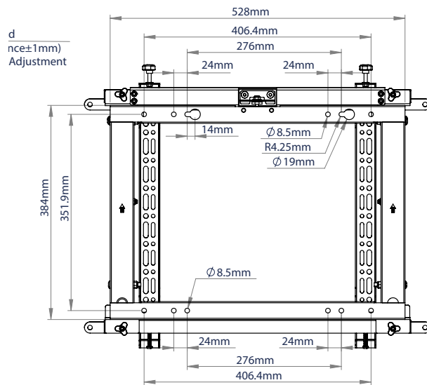
VUE ARRIÈRE
