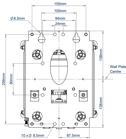
VUE ARRIÈRE AVEC BRAS ADAPTATEURS
