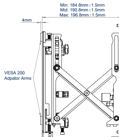
VUE LATÉRALE PROLONGÉ
