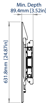
VUE LATÉRALE À PLAT CONTRE LE MUR
