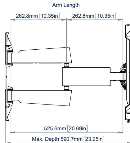
VUE LATÉRALE EXTENSION MAXIMALE
