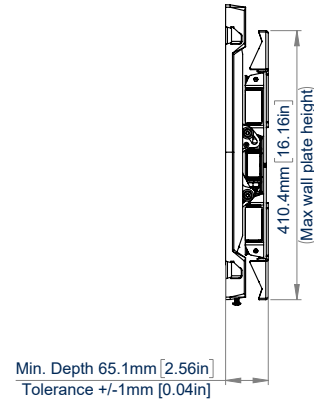
VUE LATÉRALE À PLAT CONTRE LE MUR
