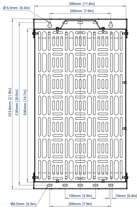
VUE AVANT PORTRAIT
