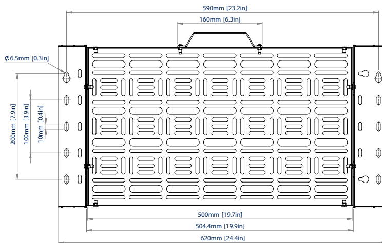
VUE AVANT PAYSAGE
