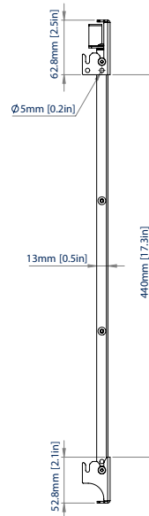
VUE LATÉRALE PORTRAIT
