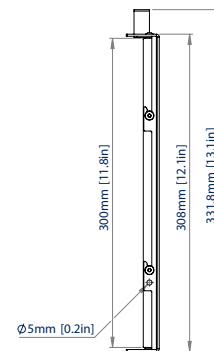
VUE LATÉRALE PAYSAGE
