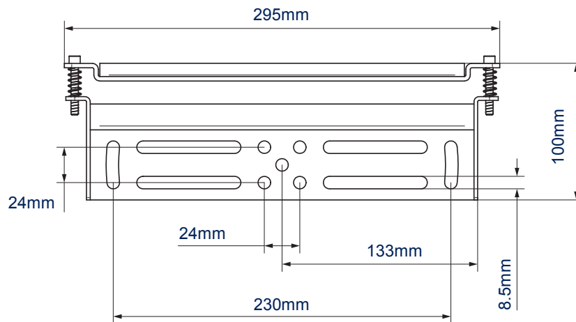
VUE DE FACE PLAQUE MURALE
