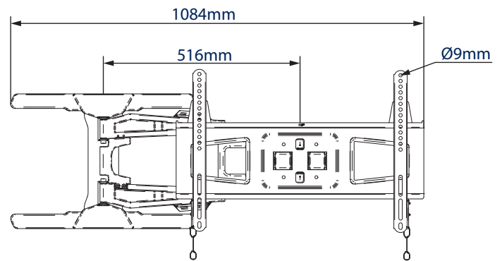
VUE DE FACE AVEC LE BRAS TENDU SUR LE CÔTÉ
