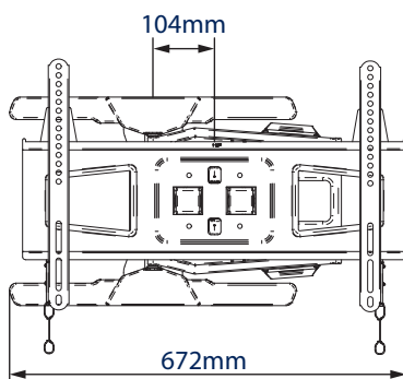
VUE DE FACE PLAT AU MUR
