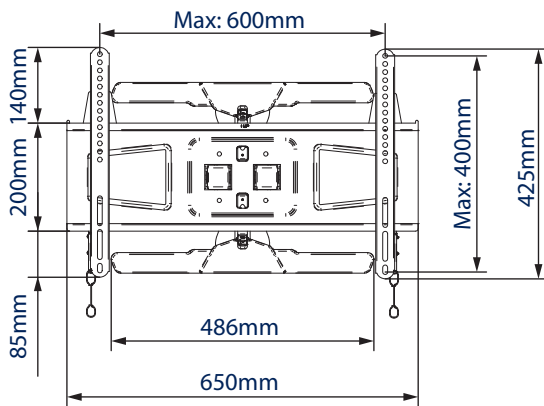
VUE DE FACE EXTENSION MAXIMALE
