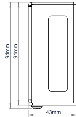
VUE LATÉRALE
