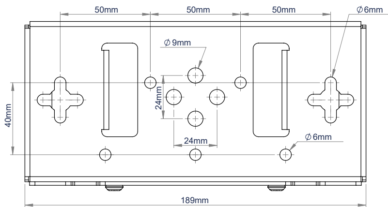
VUE ARRIÈRE
