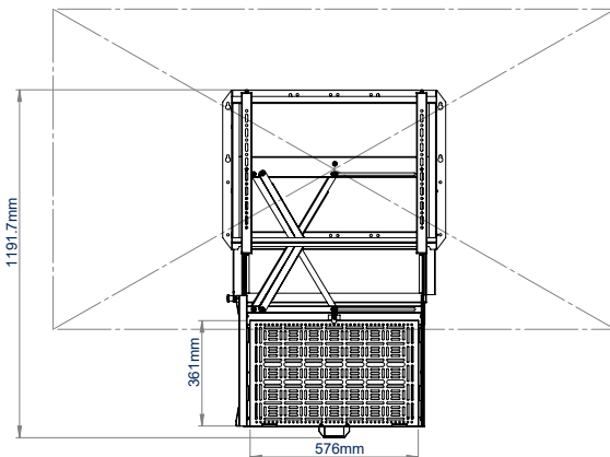
VUE DE FACE ÉCRAN DE 86" - OUVERT
