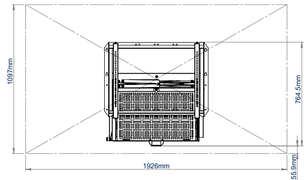
VUE DE DERRIÈRE ÉCRAN DE 86" - FERMÉ
