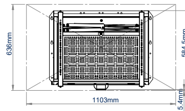
VUE DE DERRIÈRE ÉCRAN DE 49" - FERMÉ
