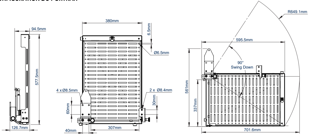
VUE LATÉRALE FERMÉE
