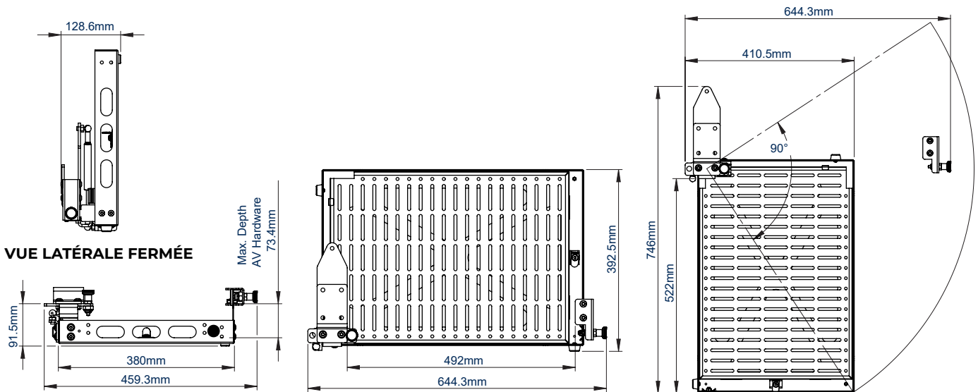
VUE INFÉRIEURE FERMÉE
