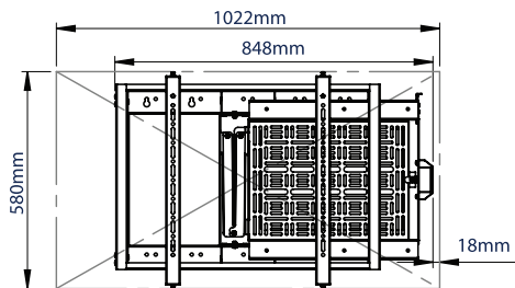
ÉCRAN 46 FERMÉ
