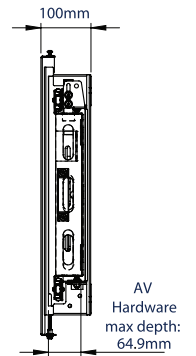
VUE LATÉRALE
