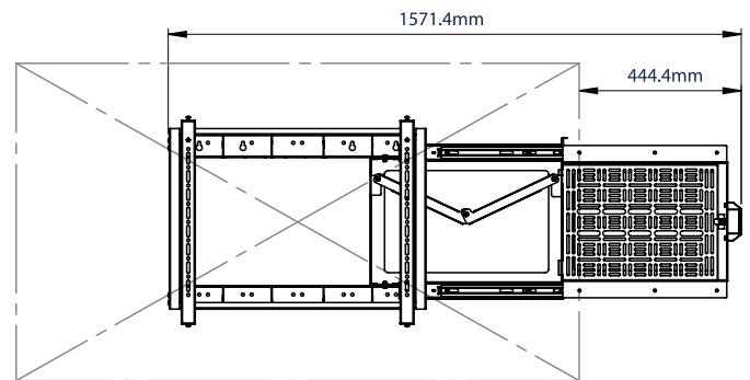
ÉCRAN 75 OUVERT
