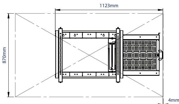
ÉCRAN 75 FERMÉ
