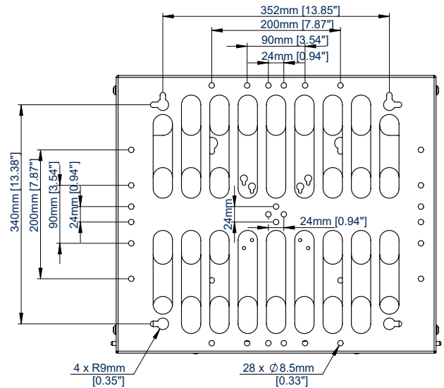
VUE ARRIÈRE
