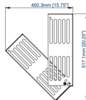
VUE LATÉRALE
