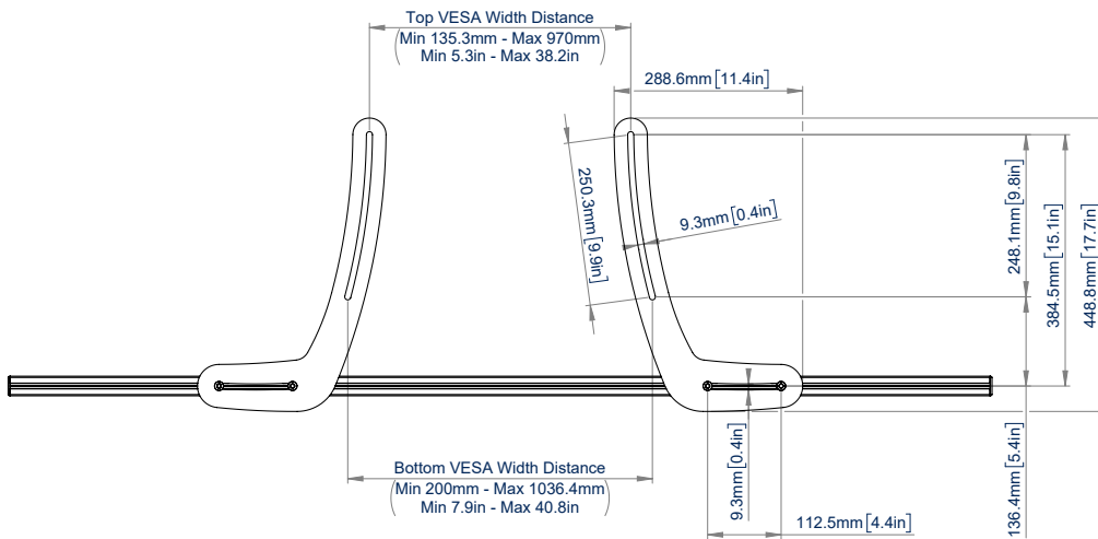
VUE ARRIÈRE
