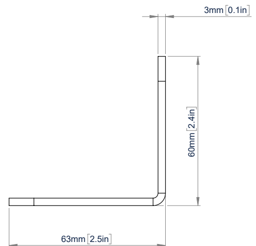
VUE LATÉRALE
