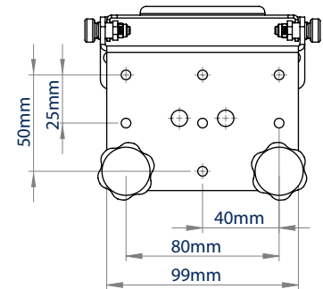
VUE ARRIÈRE
