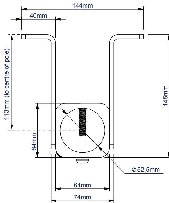
VUE TOP
